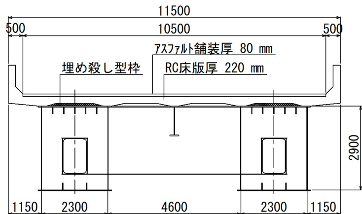
従来箱桁橋
