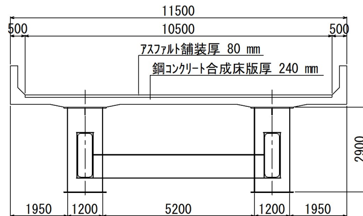
細幅箱桁橋
