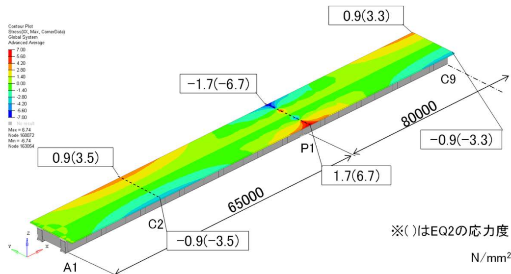
②有限要素解析(全橋 1/2モデル)
