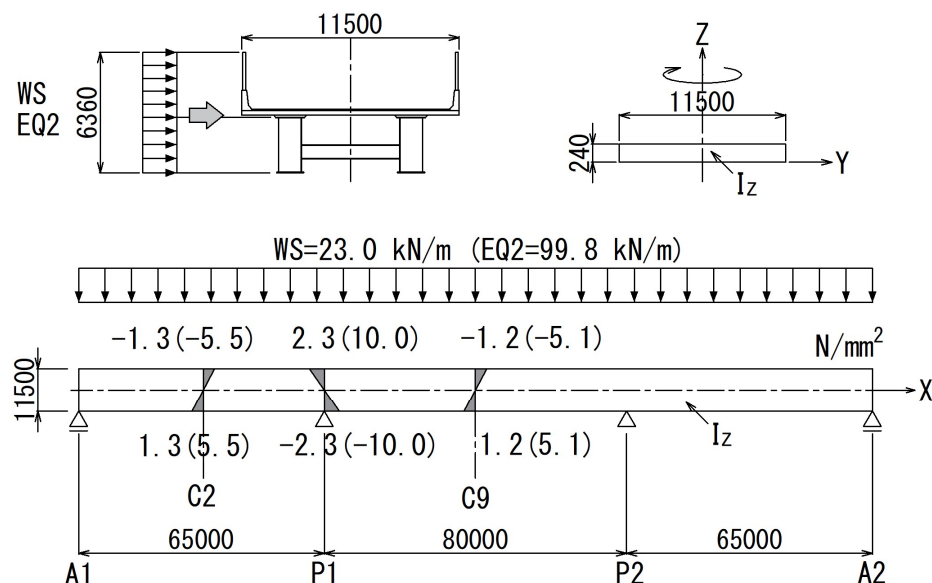
①梁モデル(床版のみ)
