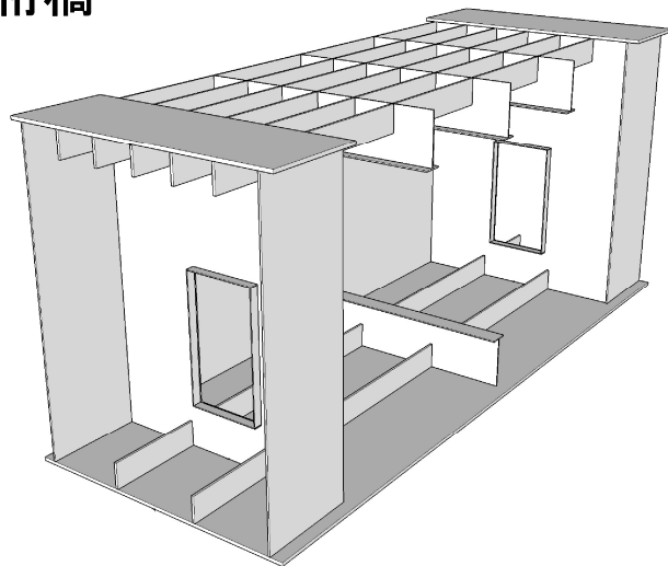
従来箱桁橋
