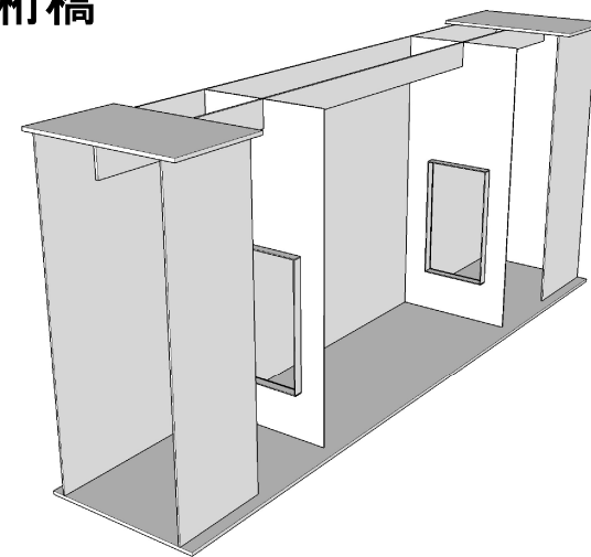
細幅箱桁橋
