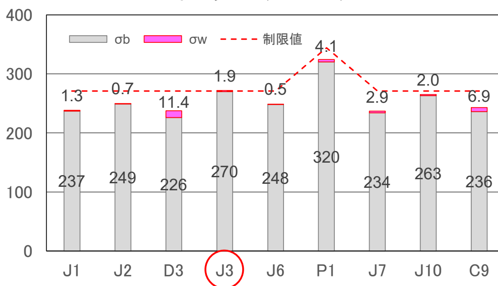
\sigma (N/mm 2 ) 下フランジ(R=300m)
