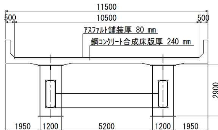
細幅箱桁橋
