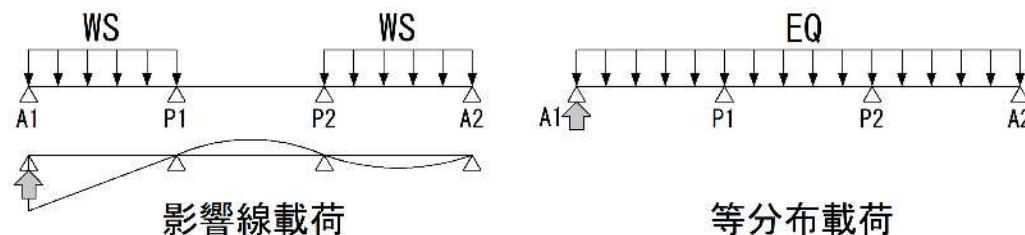
端支点(A1)の場合
