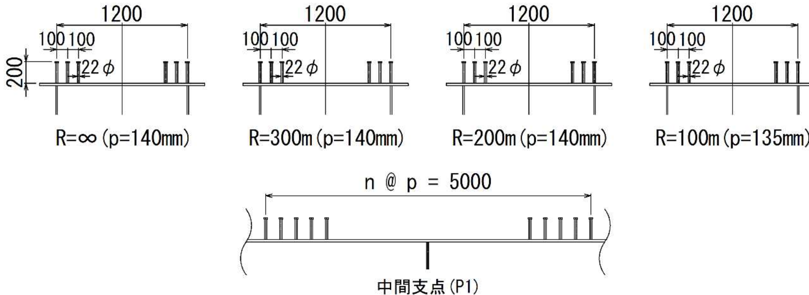
中間支点(P1): 組合せ⑪(D+EQ2)
