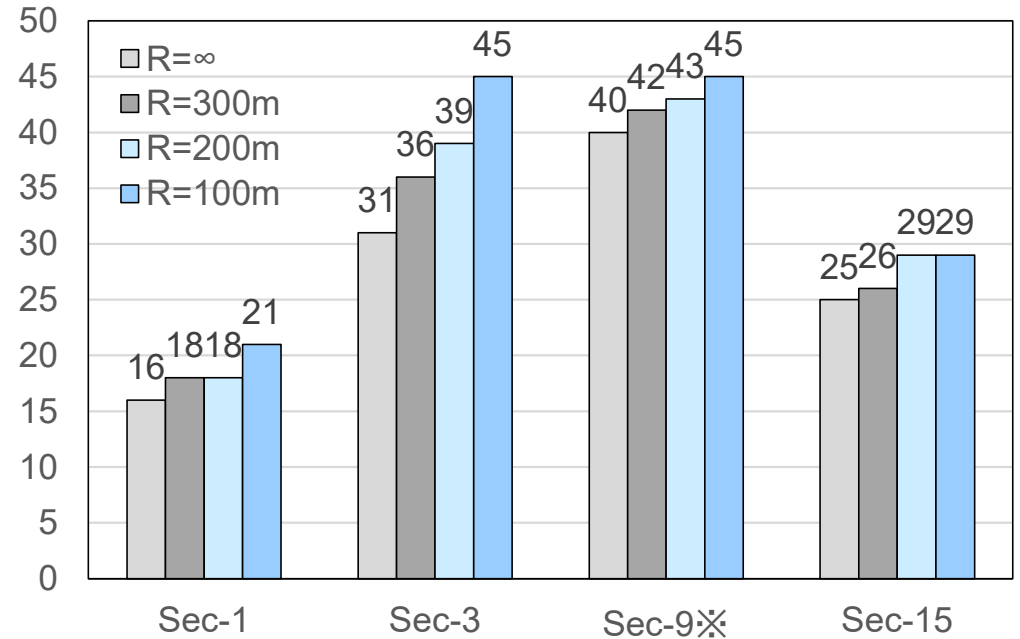
G1(外桁)下フランジ
