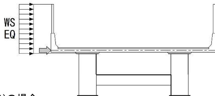
端支点(A1)の場合
