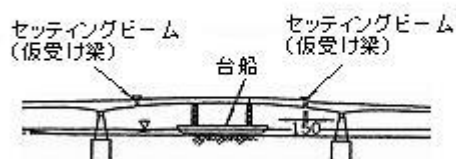
台船による一括架設
