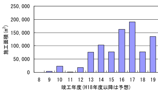
合成床版の施工実績 (Q & A より)
