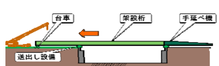
図-6 下路トラス架設桁吊り込み解体手順図
