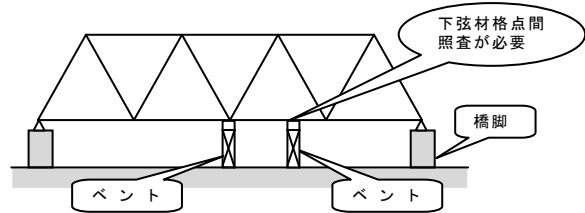
図-1 トラス橋仮受要領図
