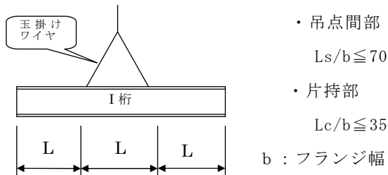
図-3 桁吊り上げ要領図
