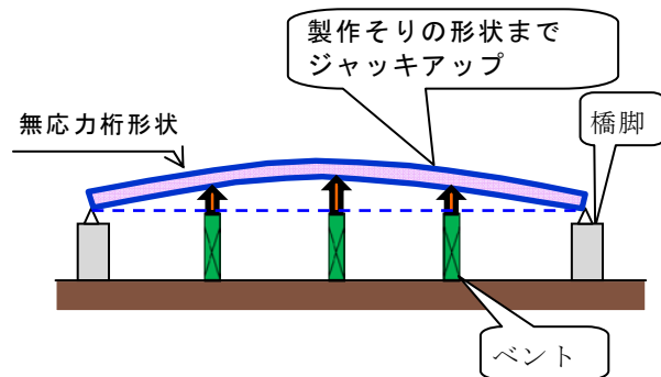
図-2 応力解放作業要領図
