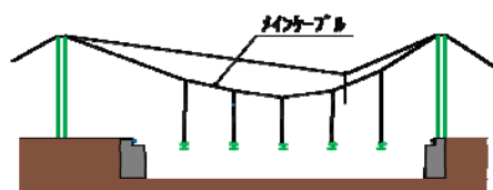
図-7 下路トラス直吊り解体手順図
