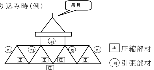
図-5 断面力発生状況図
