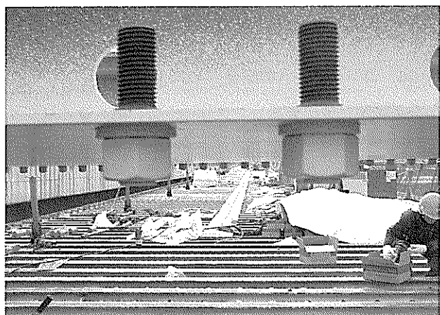
写真-34 埋殺し部節付きボルト
