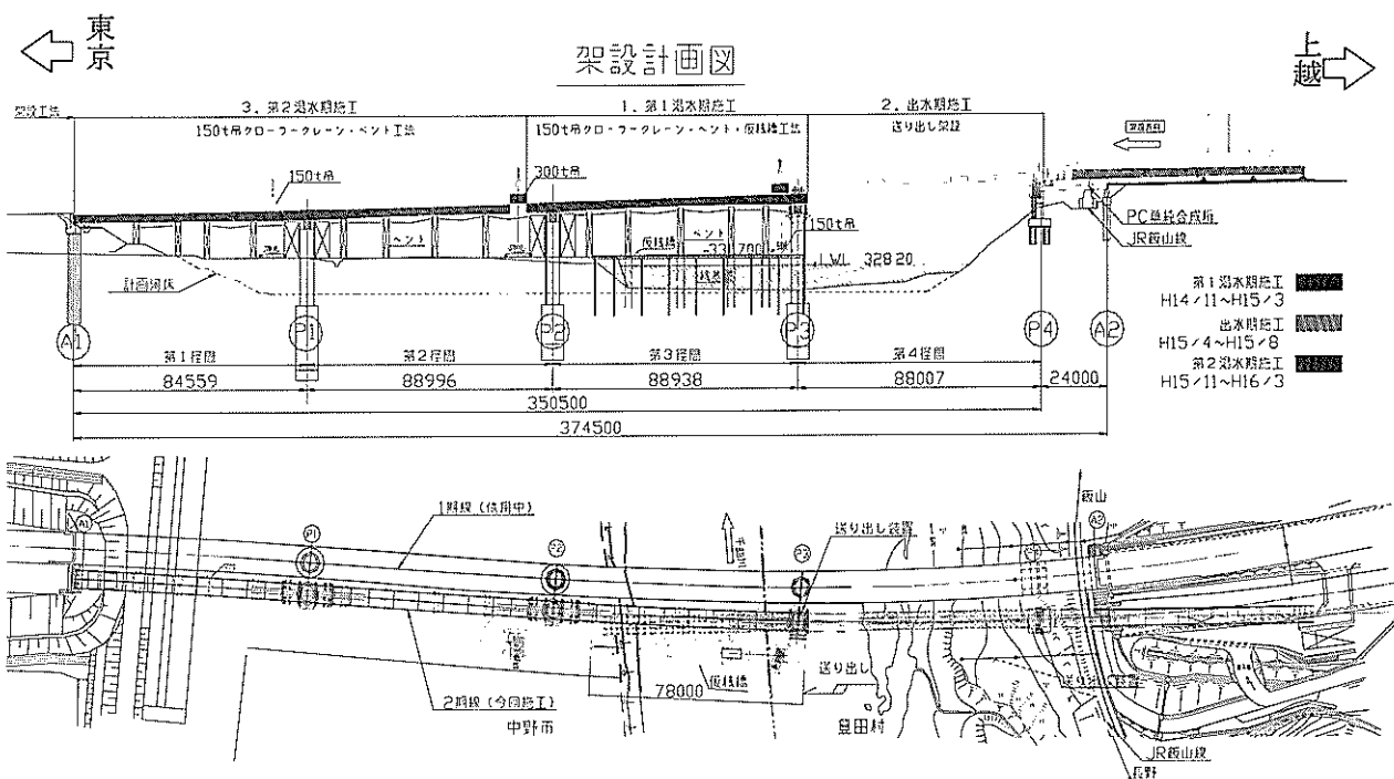
図ー8 架設計画図
