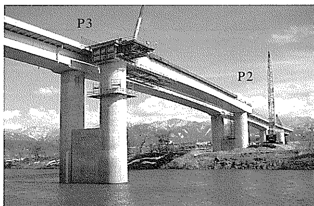
写真ー13 第3径間 (P2~P3) 架設完了
