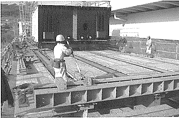
写真-24 桁縦取り状況
