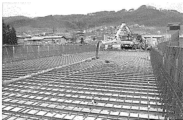
写真-41 第3,4径間配管打設
