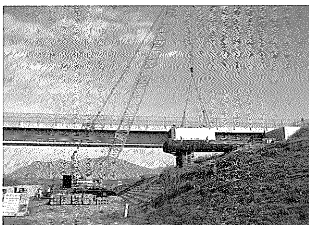
写真-23 架設状況
