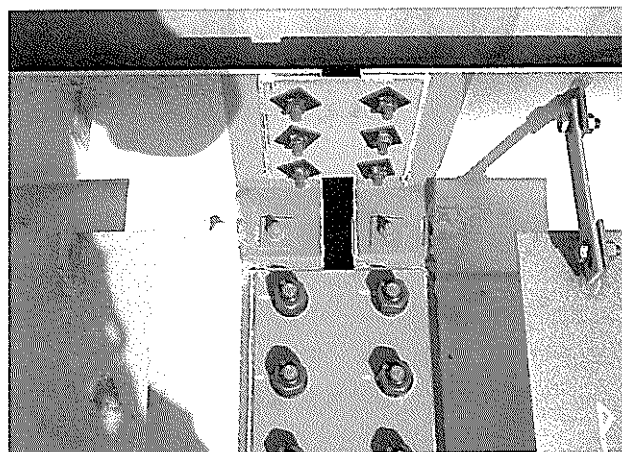
写真-33 調整パネル添接完了 張出し部TCボルト締め完了
