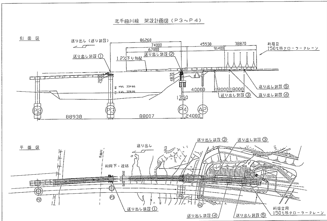
図-10 送り出し架設計画一般図
