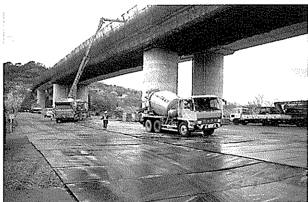
写真-40 第1,2径間ブーム打設
