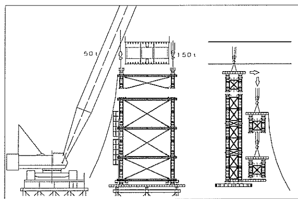
図ー9 河川ベント解体図
