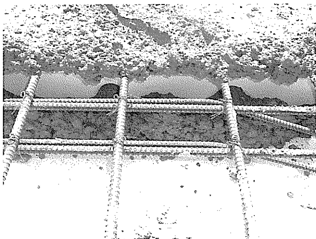
写真-43 パーフォンド孔流動状況
