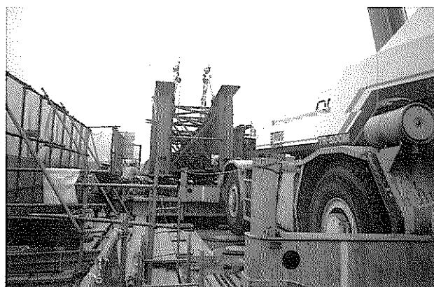
写真-21 手延べ機解体状況
