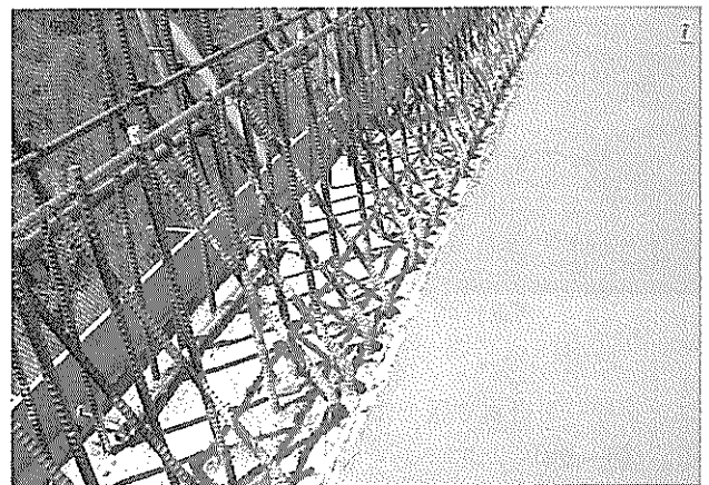
写真-45 壁高欄打継ぎ目遅延材散布完了
