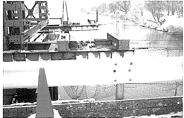
写真一15 ベント基部受け台設置状況
