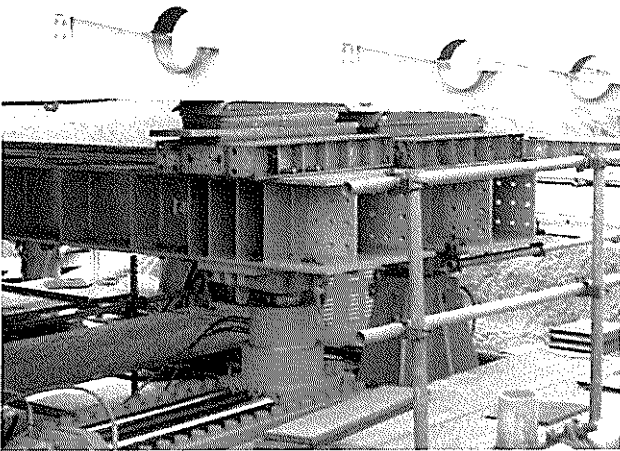
写真-29 主桁荷受点養生状況
