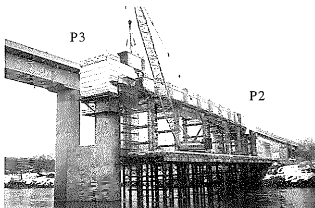
写真ー12 閉合桁の架設状況
