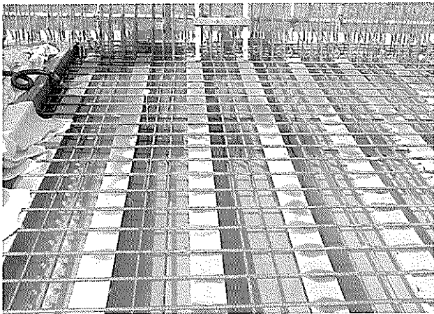
写真-48 打設前雨水滞留状況
