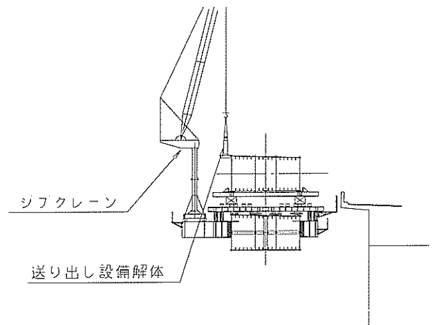
図-13 P3ジブクレーン配置図
