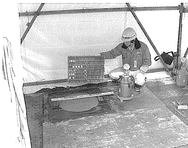
写真ー8 コンクリート受入れ検査
