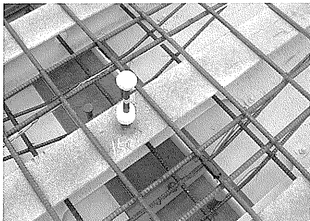
写真-42 床版厚検測棒
