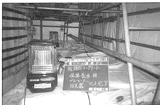
写真－10 養生設備配置完了
