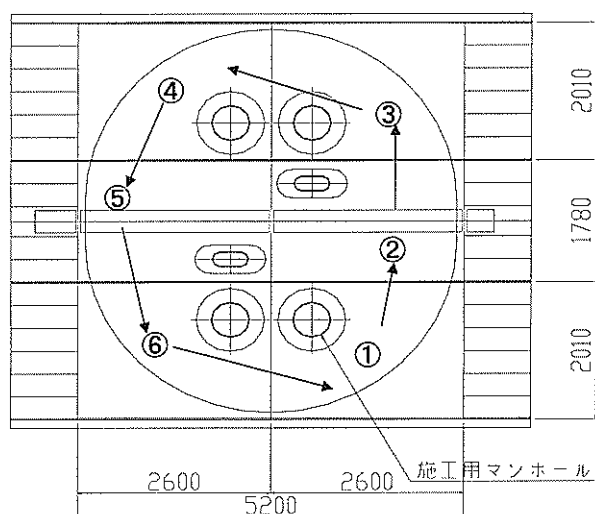
図ー7 剛結部の打込み手順
