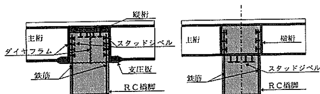
Ⅰ期線「下フランジ支圧板形式」 1) Ⅱ期線「鉄筋定着形式」
