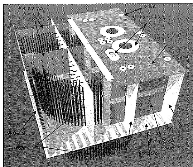
図-4 柱頭部構造概念図
