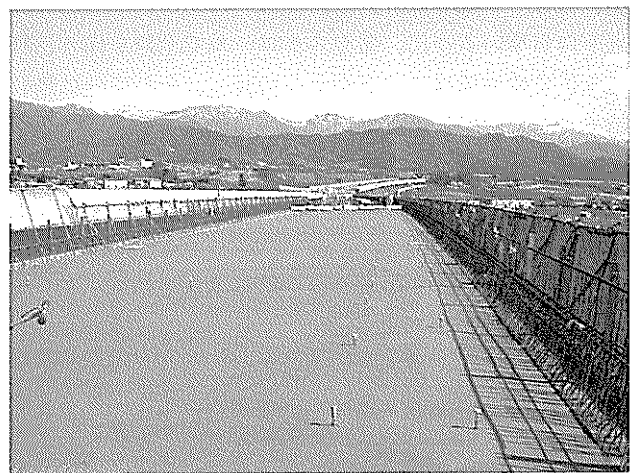
写真-46 床版打設完了
