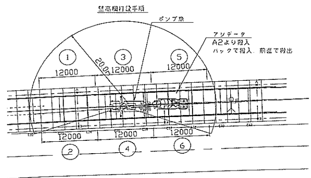
図-25 壁高欄コンクリート打込み手順
