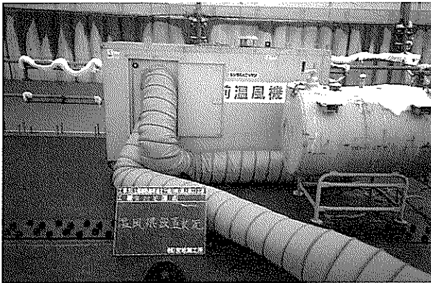
写真-28 添接部塗装用温風機設置
