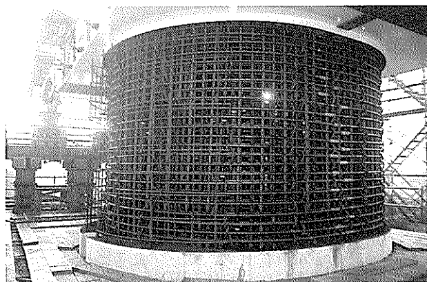
写真-1 柱頭部鉄筋の組立完了状況
