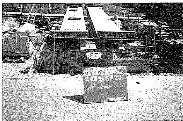
写真-17 送り出し装置配置
