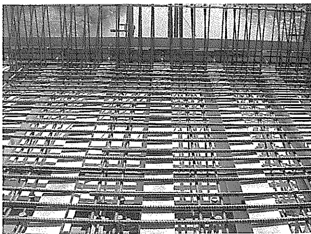
写真-39 鉄筋組立完了（支点補強部）
