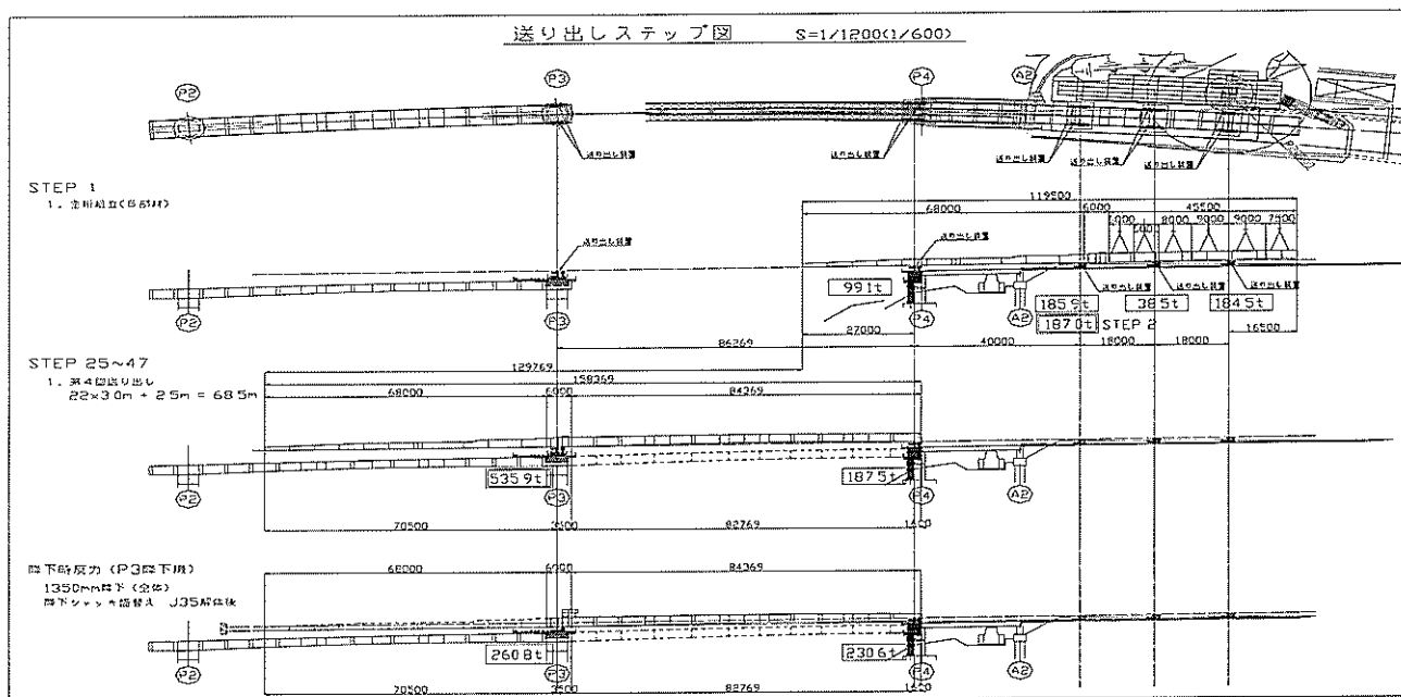
図－12 送り出しステップ図
