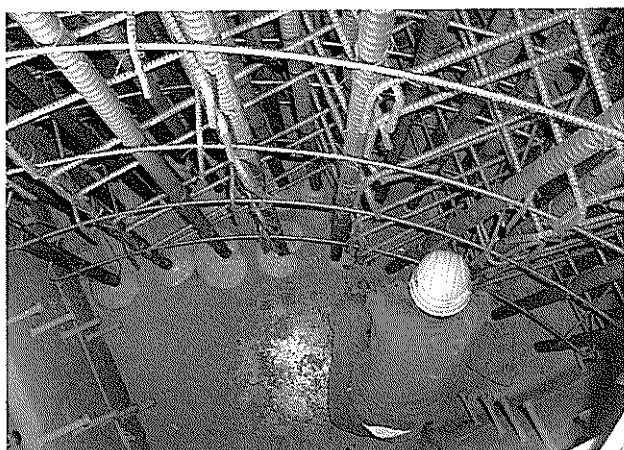
写真-3 下フランジフロー状況
