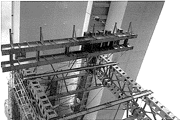
写真一14 相吊り解体状況(手前50tRC、奥150tCCで玉掛け)
