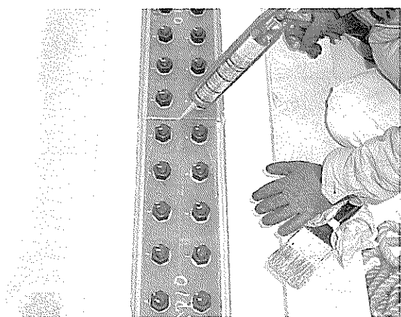
写真-35 添接部シール状況 節付きボルト本締め完了
