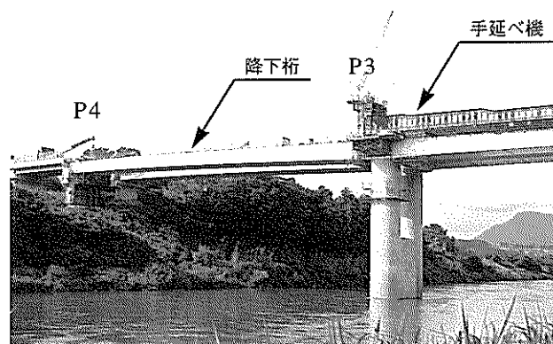
写真-20 桁降下完了
