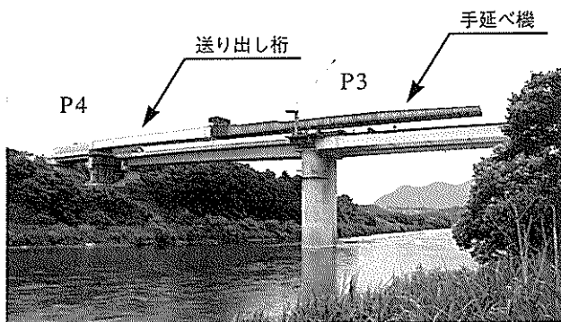
写真-16 送り出し状況
