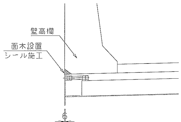
図-26 壁高欄・側板継ぎ目シール位置
