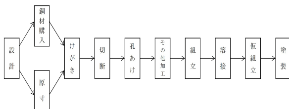
図-1 鋼橋工場製作の流れ
