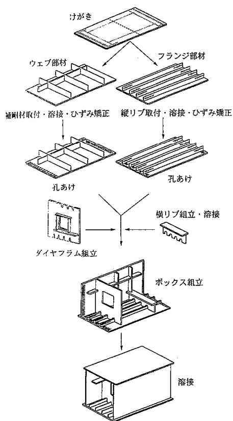
図-3 箱桁パネル工法フロー図 6)
