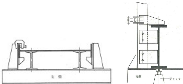
図-2 部材の組立治具の例 6)
