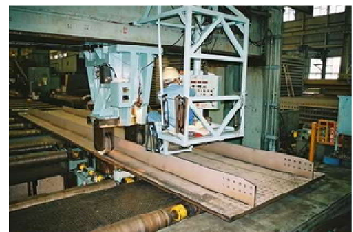
写真-15 パネル矯正機
