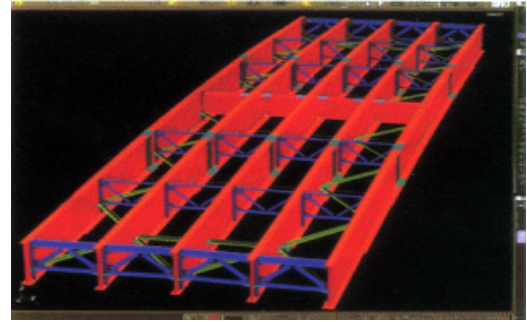
写真-28 シミュレーション仮組立実行画面
