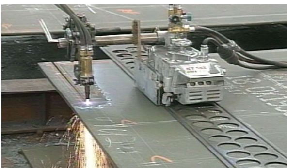
写真-5 ポータブルガス切断
