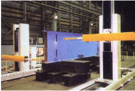
写真-26 3次元視覚センサーによる計測 5)
