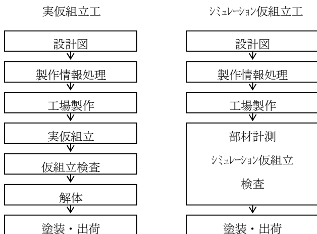
図-4 仮組立工法別による工程比較
