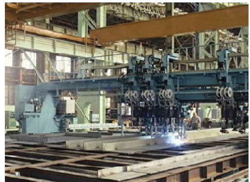
写真-14 縦リブ組立装置
